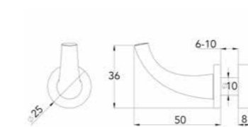
PSG0103 Coat Hook
