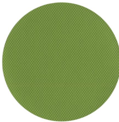
MN 21953
